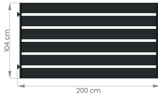
Przęsło nowoczesne:
