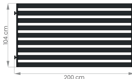
Przęsło nowoczesne:
