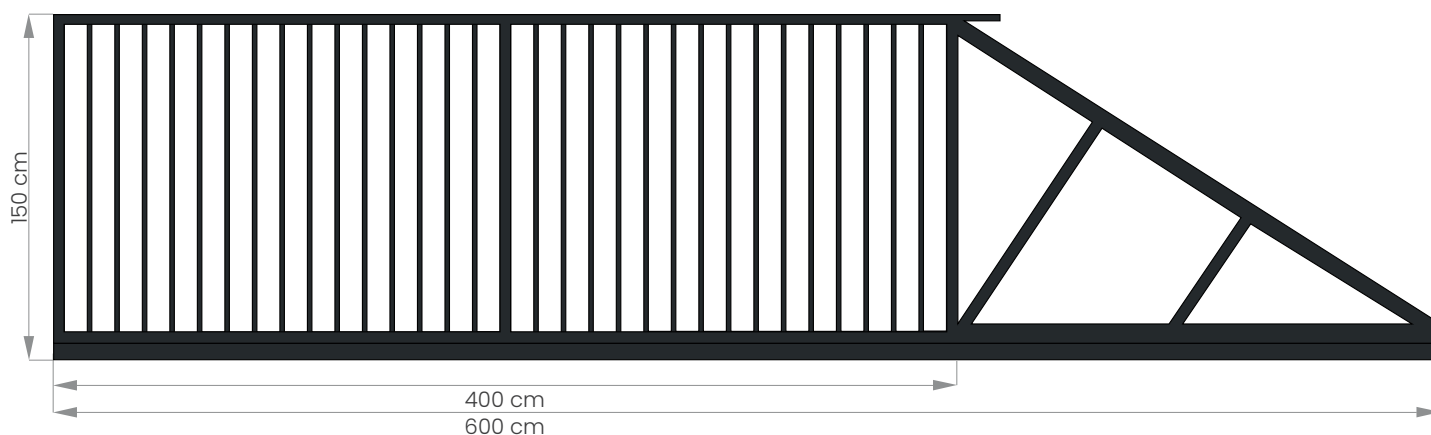
Brama przesuwna nowoczesna:
