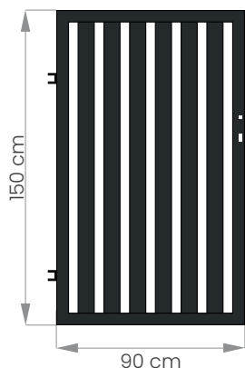
Furtka nowoczesna:
