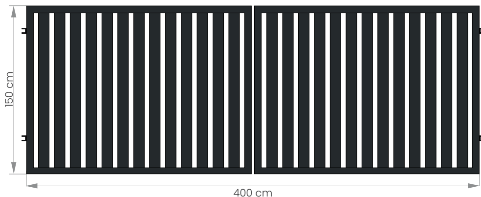
Brama dwuskrzydłowa nowoczesna:
