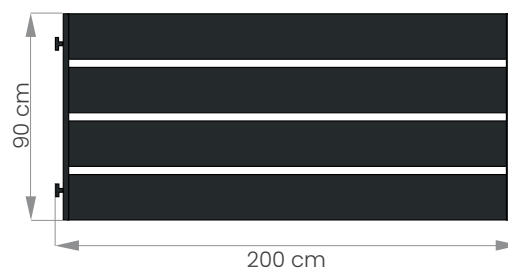
Przęsło nowoczesne:
